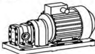
Общий вид насосного агрегата БГ11-2 с двигателем
