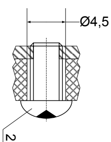
A-A (2:1)
