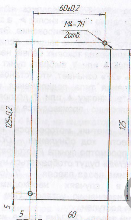
Рисунок 5 – Разметка панели для заднего присоединения проводов РДЦ-01-055, РДЦ-01-205
