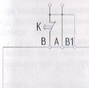
Рисунок 4 – Схема электрическая принципиальная реле ВС43-3
