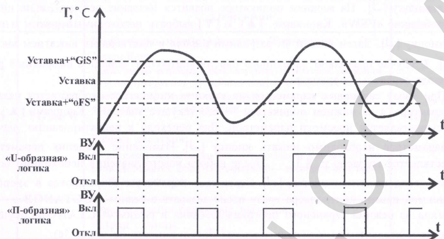
Рисунок 7: Пример работы ЛУ в режиме «П-образной» и «У-образной» логики.
