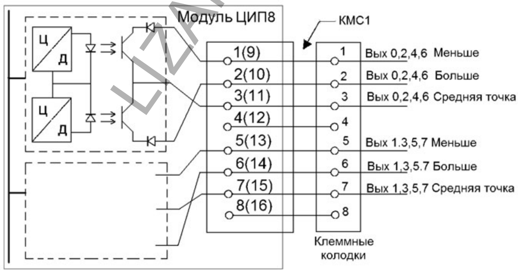
Рисунок 3 – Модуль цифро-импульсного преобразования ЦИП8. Схема внешних подключений
