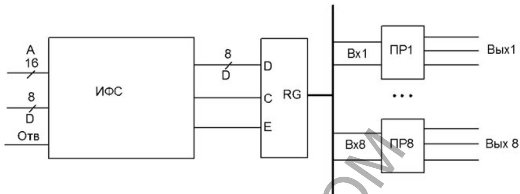
Рисунок 3 – Модуль цифро-импульсного преобразования ЦИП8. Схема структурная.
