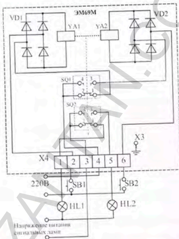
Рисунок В.2 - Исполнение электромагнита с сальниковым вводом
