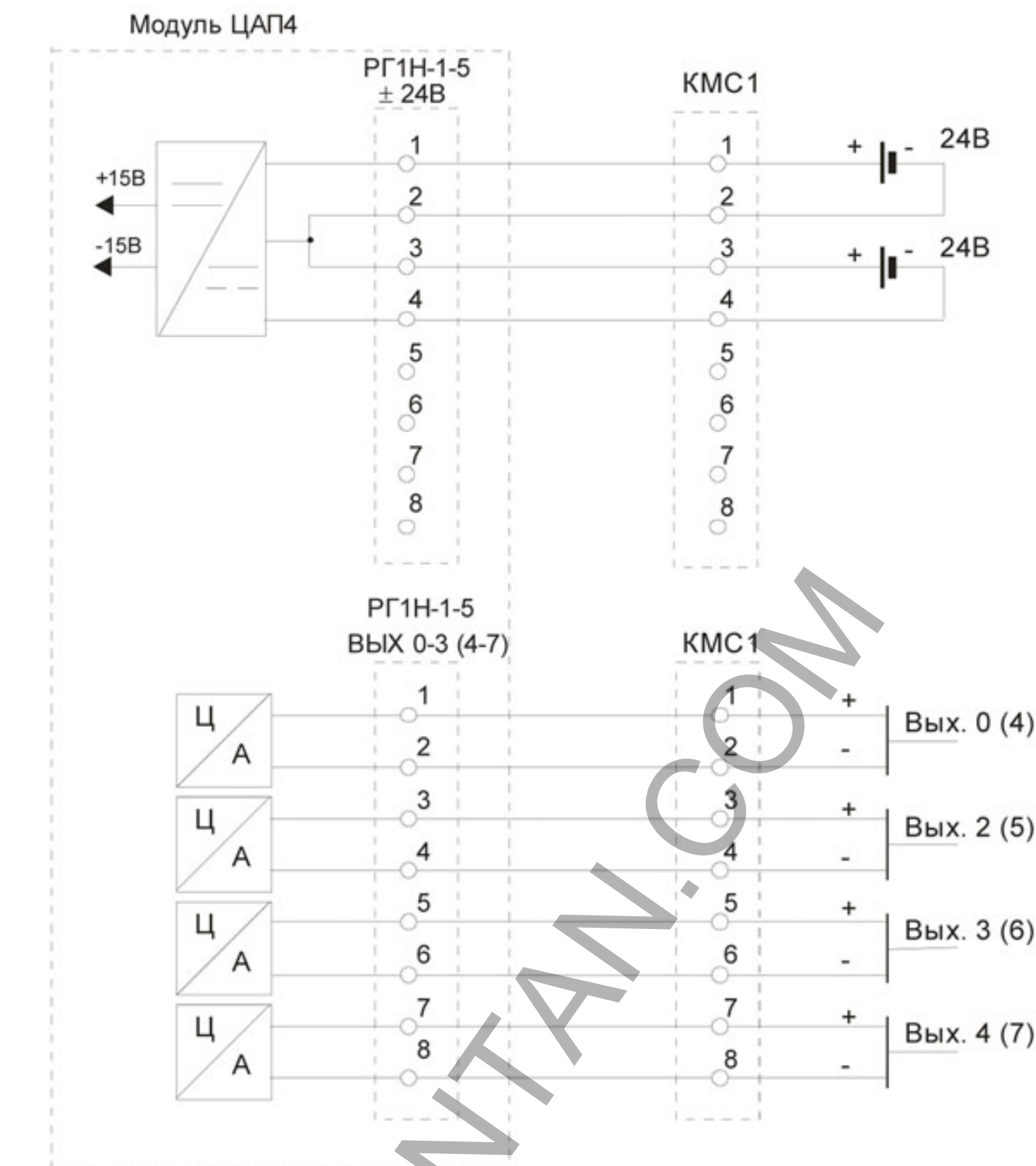
Рисунок 4 – Модуль цифро-аналогового преобразования ЦАП4. Схема внешних подключений
