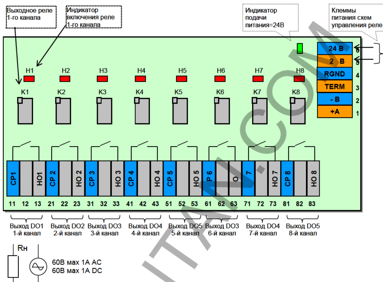
Рисунок Б.3.4- расположение сигналов и баритные размеры клеммно-блочного соединителя КБЗ-30К-11
