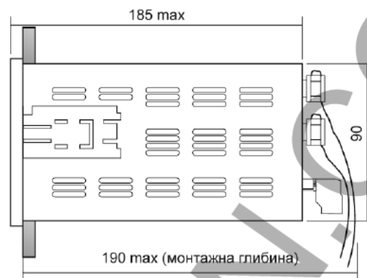
Рисунок А.1 - Габаритные и присоединительные размеры
