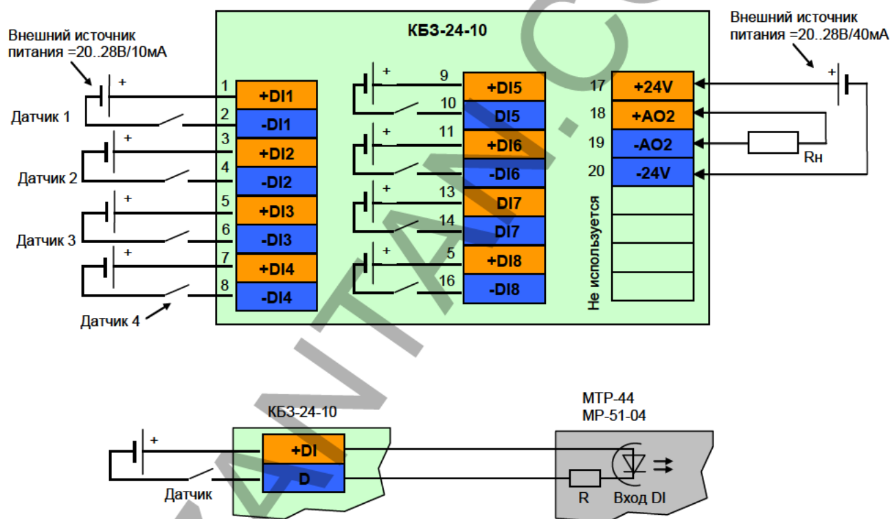
Рисунок Б.3. 2 - Подключение сигналов модуля расширения МР-51-04 с помощью клеммно-блочного соединителя KB3-24-10
