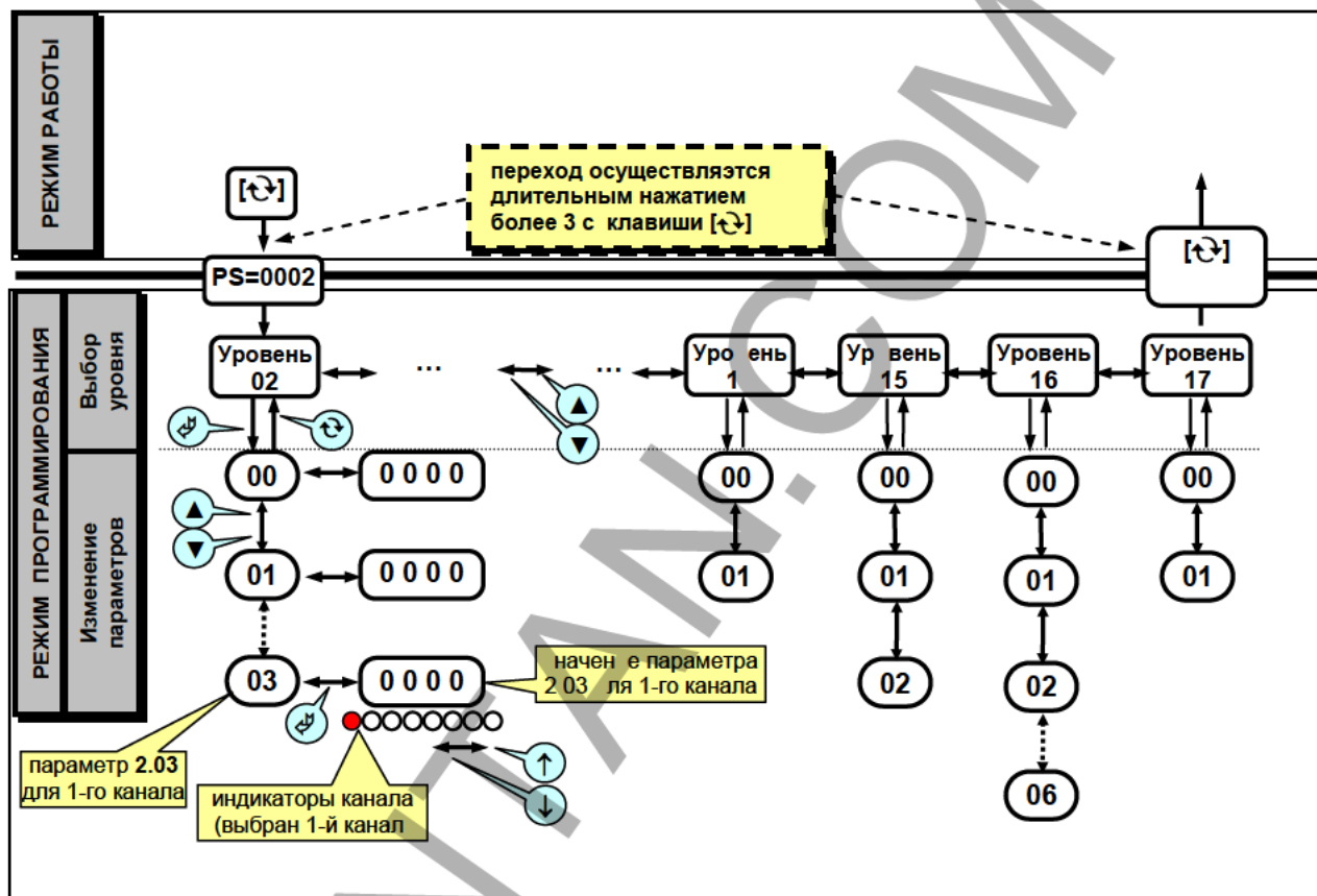
Рисунок 6. - Диаграмма уровней конфигурации и настроек
