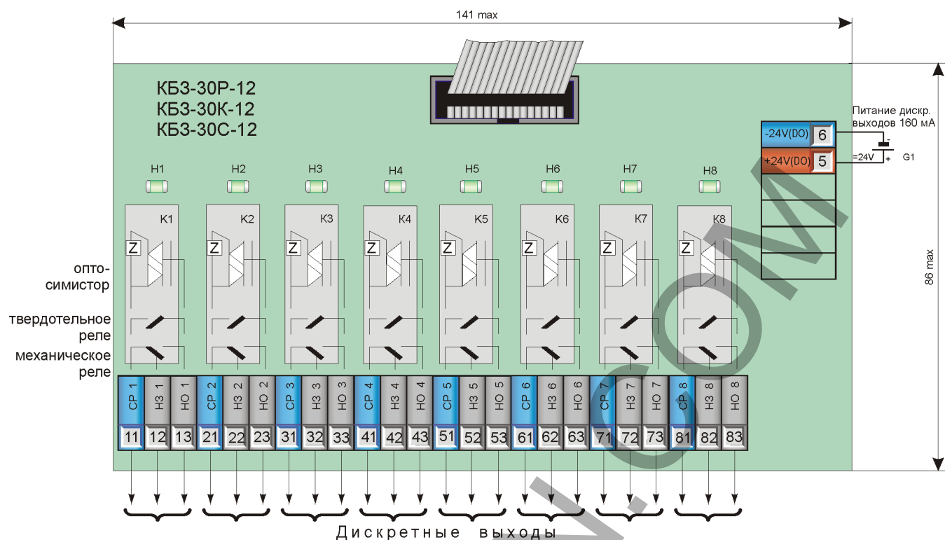
Рисунок Б.3.11 - Подключение сигналов в модуль расширения МР-51-03 с помощью клеммно-блочного соединителя КБ3-30-12, КБ3-30К-12, КБ3-30С-12
