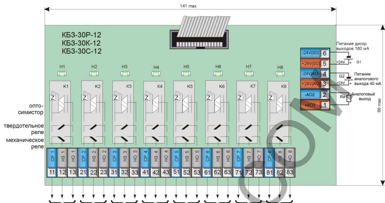
Рисунок Б.3.16 - Подключение сигналов модуля расширения МР-51-06 с помощью клеммно-блочного соединителя КБ3-30P-12, КБ3-30C-12, КБ3-30K-12
