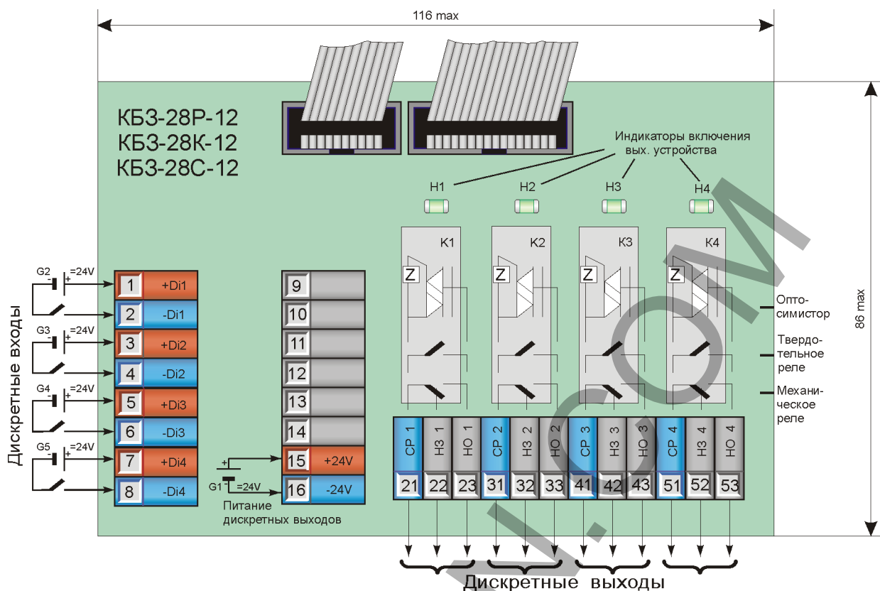
Рисунок Б.3.9 – Подключение сигналов модуля расширения МР-51-02 с помощью клеммно-блочного соединителя КБ3-28Р-12 КБ3-28С-12, КБ3-28К-12
