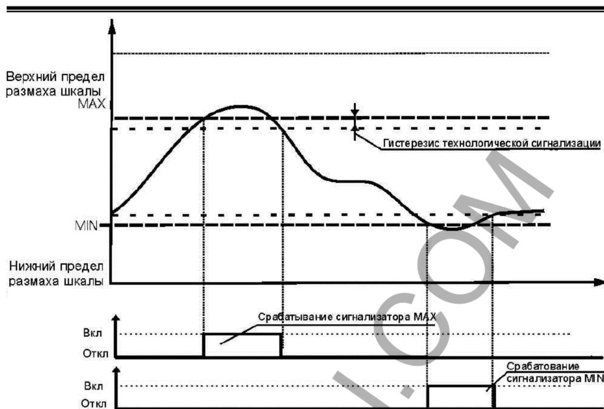
Рисунок В.4 - График срабатывания абсолютной технологической сигнализации
