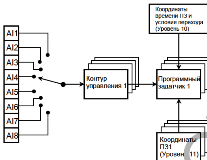
Рисунок 5.7 - Структурная блок-схема работы программного датчика
