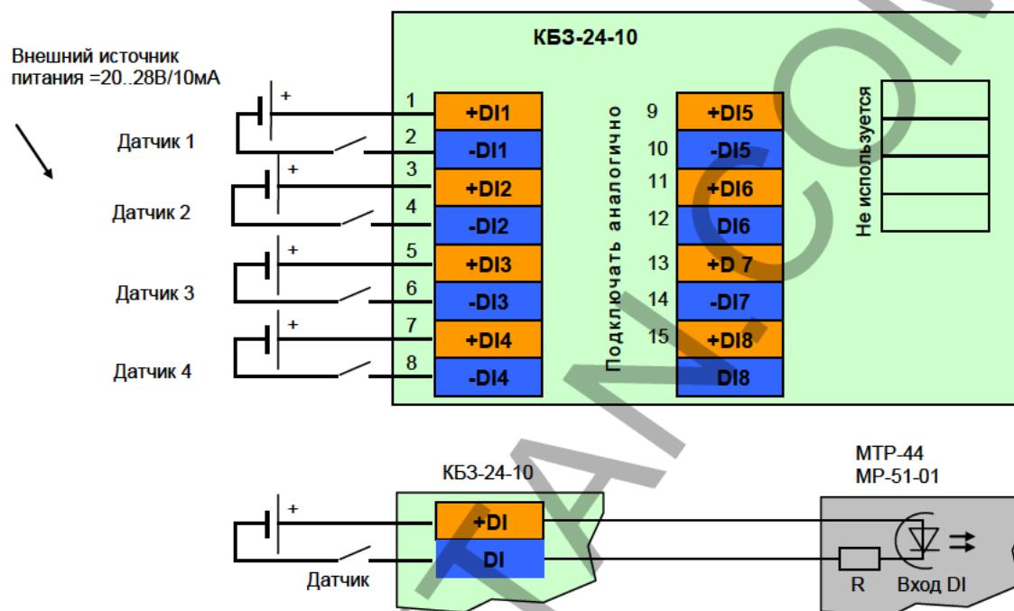
Рисунок Б.3.7 - Подключение сигналов модуля расширения МР-51-01 с помощью клеммно-блочного соединителя КБ3-24-10
