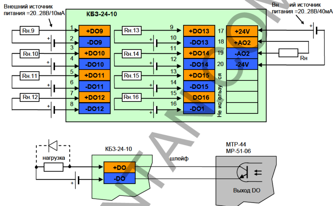
Рисунок Б.3.15 Подключение сигналов модуля расширения МР-51-06 с помощью клеммно-блочного соединителя KB3-24-10
