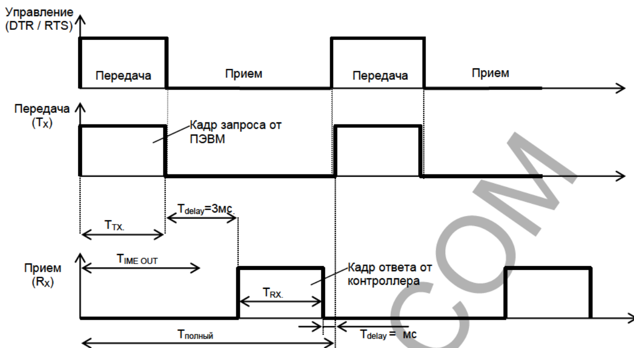
Рисунок 7.1. Временные диаграммы управления передачей приемом блока интерфейсов БПИ-485.
