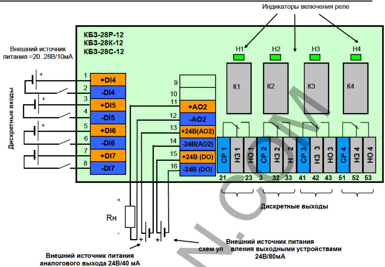
Рисунок Б.3.14 - Подключение сигналов в модуль расширения МР-51-05 с помощью клеммно-блочного соединителя КБ3-28Р-12, КБ3-28С-12, КБ3-28К-12
