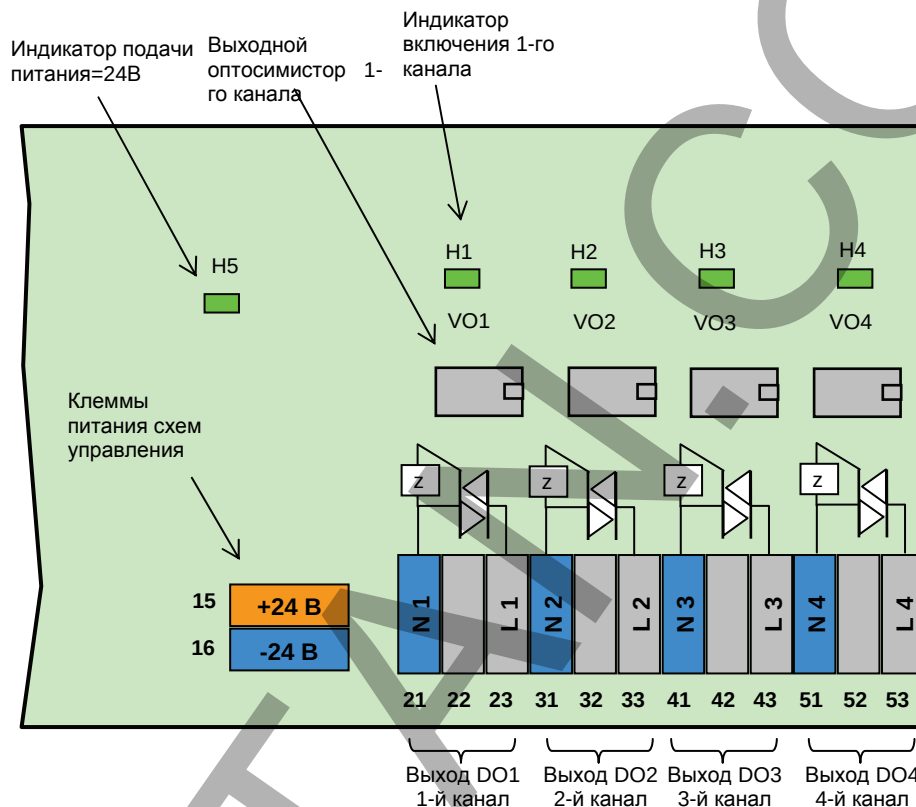
Рисунок Б.18 - Подключение дискретных нагрузок с помощью КБ3-28С-11
