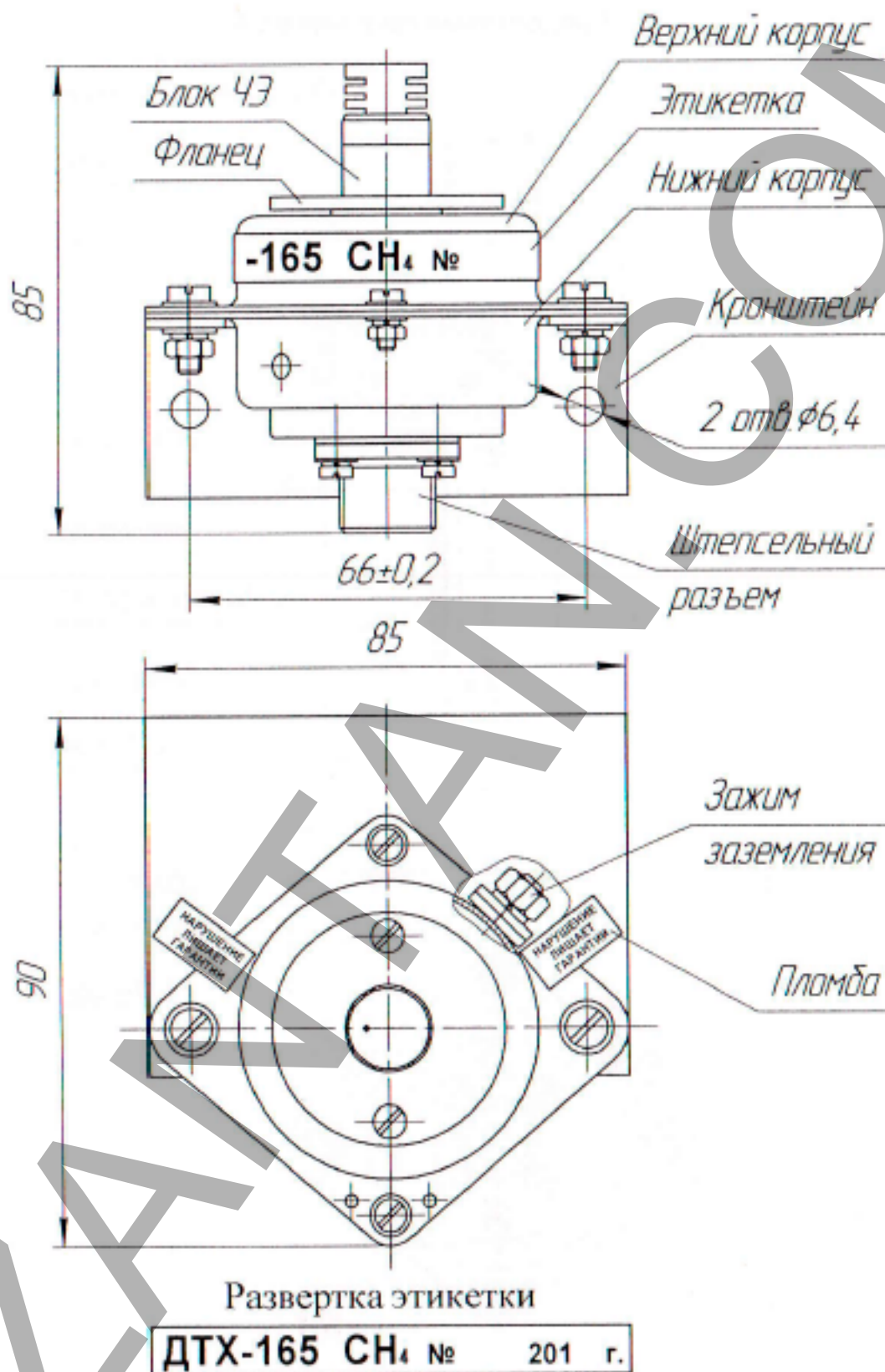
Рисунок А.4 – Общий вид датчика ДТХ-165
