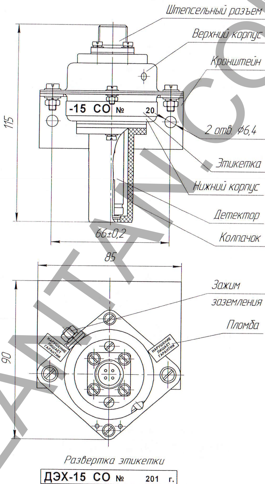
Рисунок А.5 – Общий вид датчика ДЭХ-15
